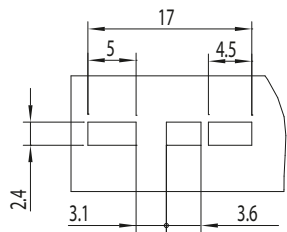
MICROCON SMDP 1P
