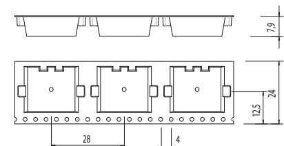
MCC SMDP 3P REEL
