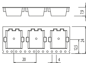
MCC SMDP 2P REEL
