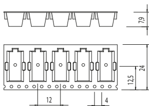
MCC SMDP 1P REEL
